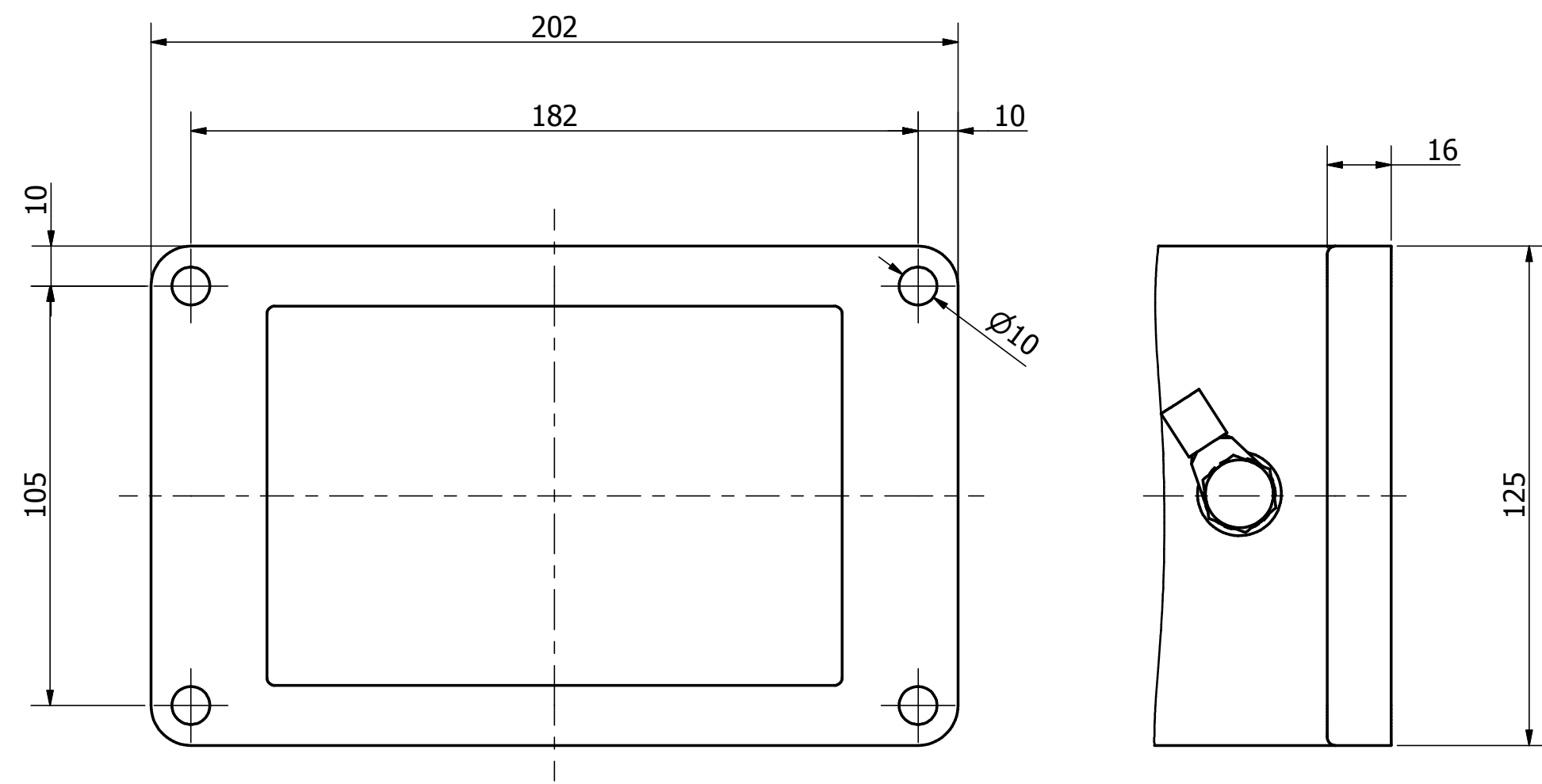
VIEW A-A ( 2 : 3 )
